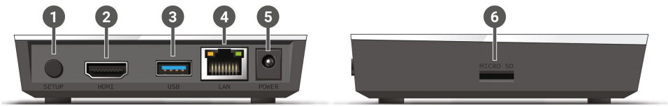
Abbildung 1: Anschlüsse
