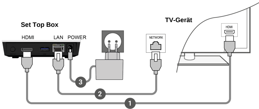
Abbildung 3: Kabelverbindungen
